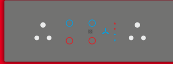
8M4S1F2Skt-4 Switch 1 Fan 2 Socket
